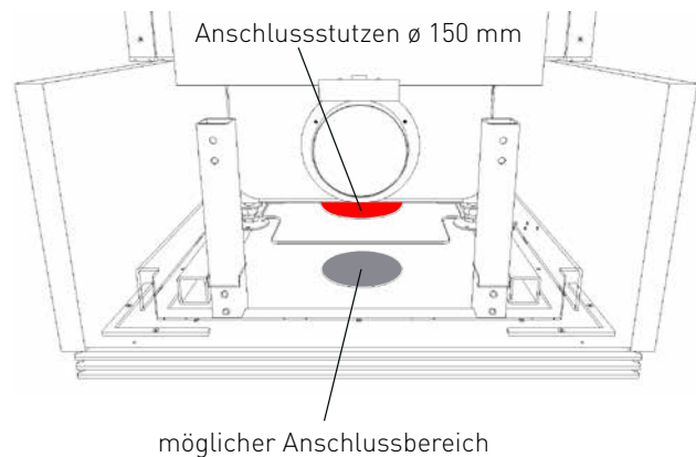
Perspektive Anschlusssituation unten
