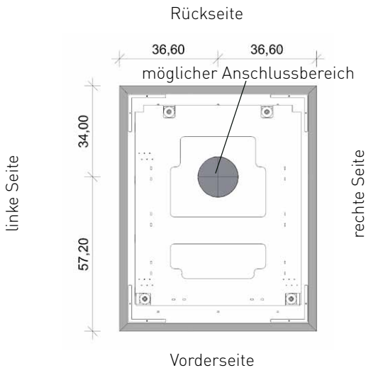
Draufsicht der Sockelplatte
