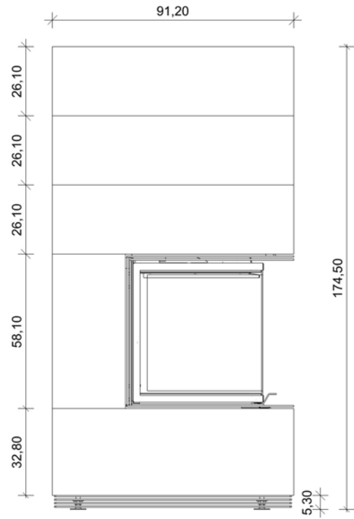
Ansicht linke Seite
