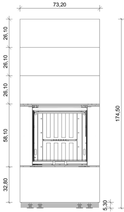
Ansicht Vorderseite
