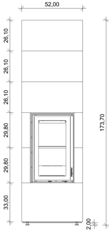
Ansicht Vorderseite
