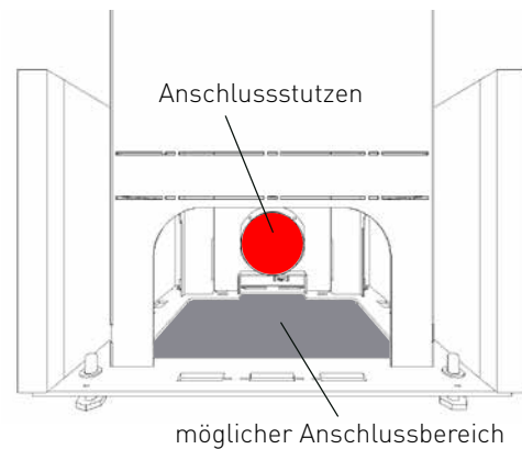
Perspektive Anschlusssituation unten
