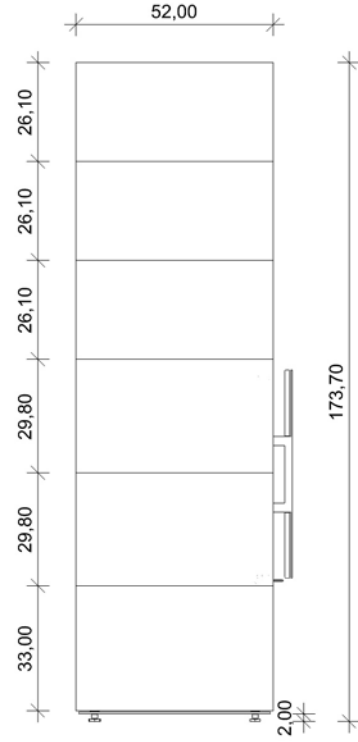
Ansicht linke Seite
