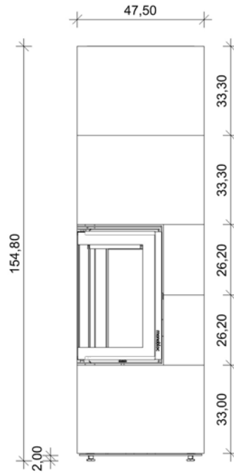
Ansicht rechte Seite
