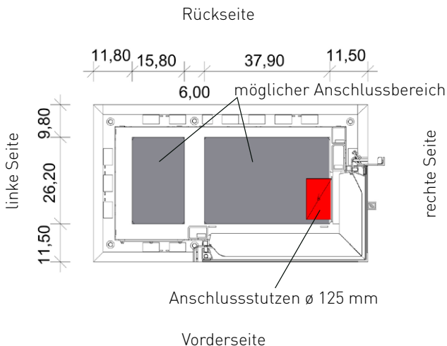
Draufsicht der Sockelplatte
