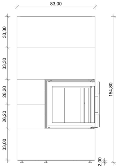
Ansicht Vorderseite
