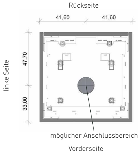
Draufsicht der Sockelplatte
