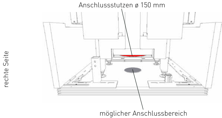
Perspektive Anschlusssituation unten
