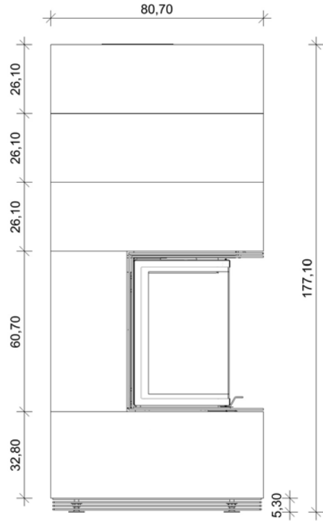
Ansicht linke Seite
