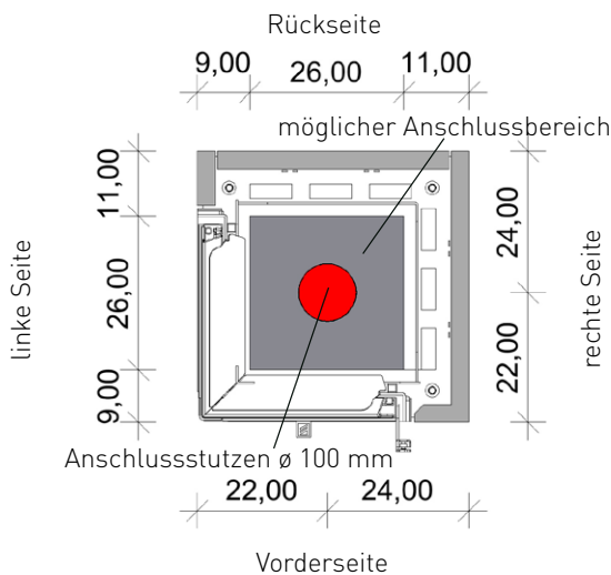
Draufsicht der Sockelplatte
