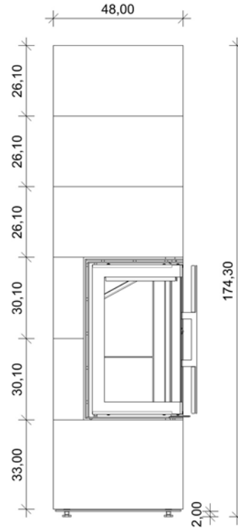
Ansicht linke Seite
