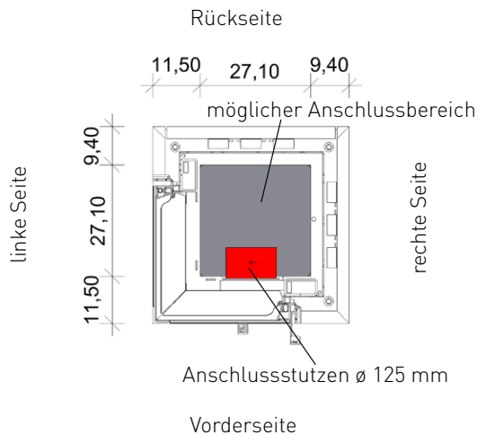
Draufsicht der Sockelplatte
